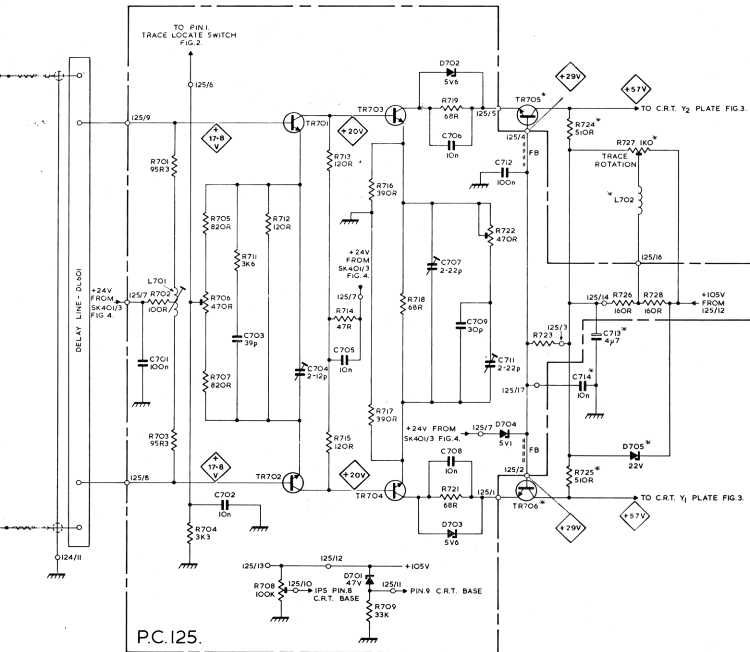
MAIN 'Y' AMPLIFIER - D83 FIG. I.
