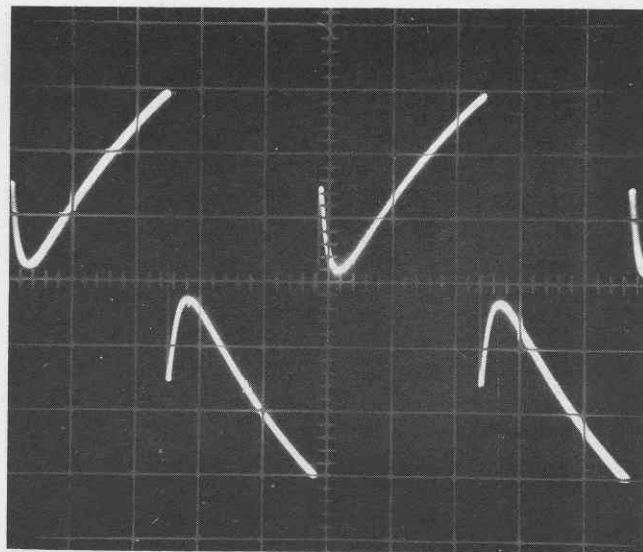
Fig. 38 Crystal Phono Input
