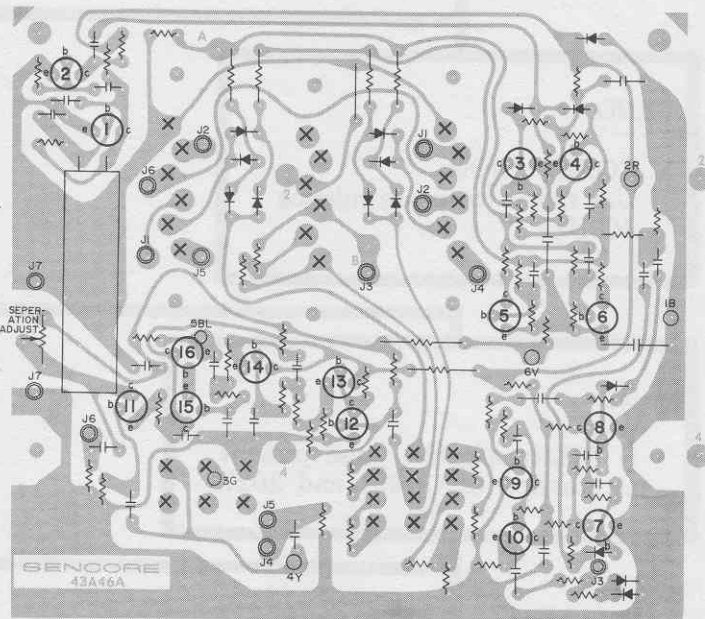
Fig. 70B Foil Side
