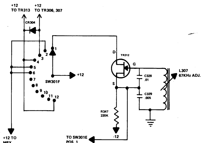
Fig. 58 67KHz Oscillator
