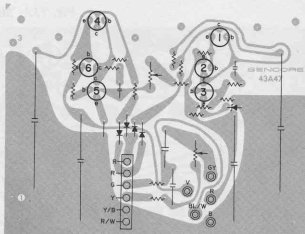
Fig. 73B Foil Side
