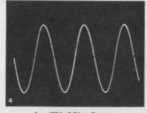
4. 400Hz, 2.5V p-p Sine wave
