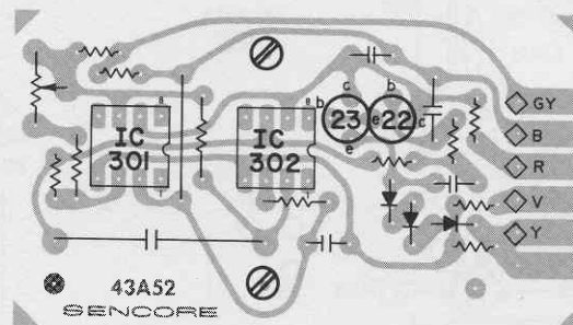
Fig. 72B Foil Side
